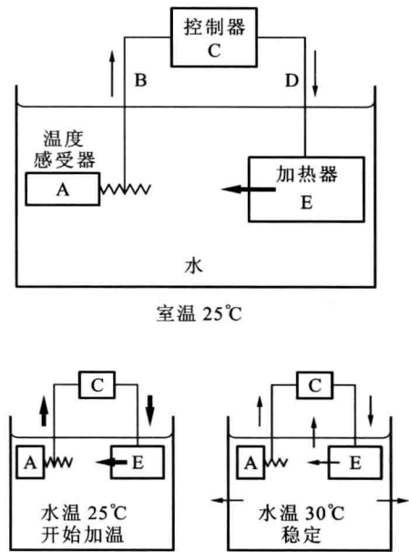
图 6.13 恒温水浴的水温控制
