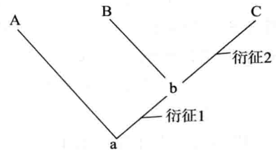
图27.10 分支系统与衍征 物种A、B、C是三个现生的近缘种。在把握了它们之间一致的和分异的性状之后,衍征1为物种B、C的共衍征,而物种A没有这个特征,据此将物种B-C和物种A分为二个姐妹分支。衍征2是物种C的独征,据此可判断物种B和C是从共同祖先物种b分开来的姐妹分支。
