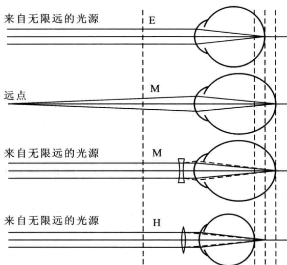
图 14.6 眼的折光异常及其矫正(仿自Ruch,1960) E. 正常眼。M. 近视眼。H. 远视眼。虚线表示矫正透镜的作用。
