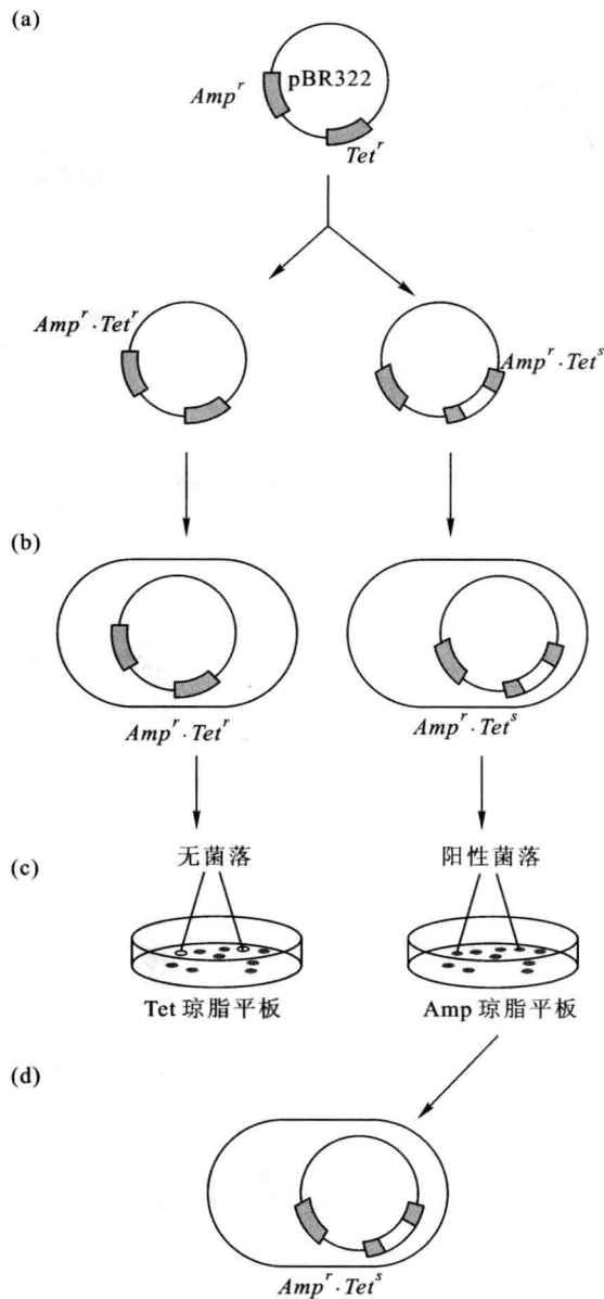
图 23.6 应用插入失活分离转化子 (仿自吴乃虎, 1998)
