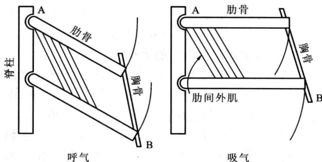
图 9.5 胸式呼吸时肋骨位置的变化
