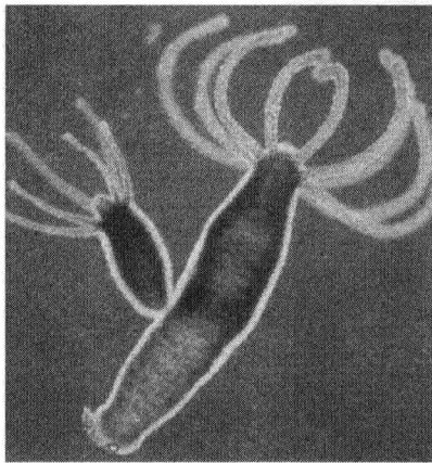
图 16.2 水螅出芽(引自 Purves,1998)
