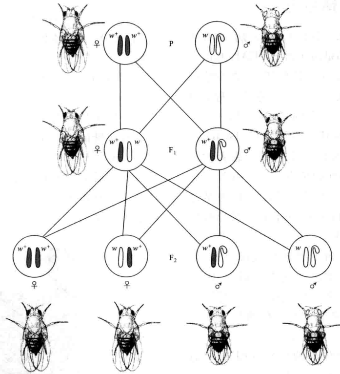
图 20.9 果蝇白眼的伴性遗传分析
