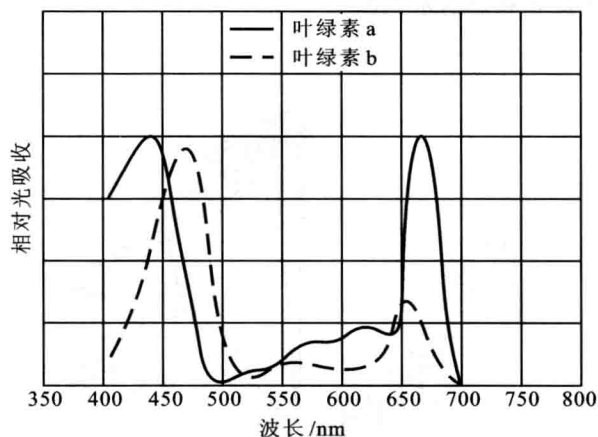
图 4.23 叶绿素 a 和 b 的吸收光谱
