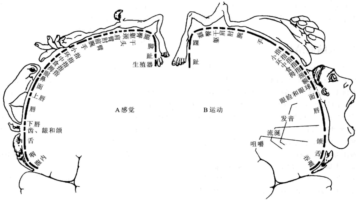
图 13.20 大脑皮质运动区和体觉区与躯体各部分的关系(仿自 Penfield,1950)
