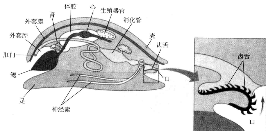
图 32.11 软体动物的基本结构 (仿自 Campbell 等, 2000) 图示真体腔和完整的消化管, 齿舌是一种可以往复运动的锉状结构, 可将食物刮成小片。
