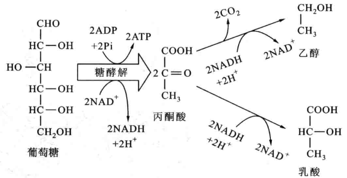
图 4.19 乙醇发酵和乳酸发酵
