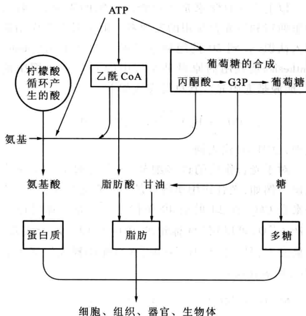
图 4.21 生物大分子合成示意图
