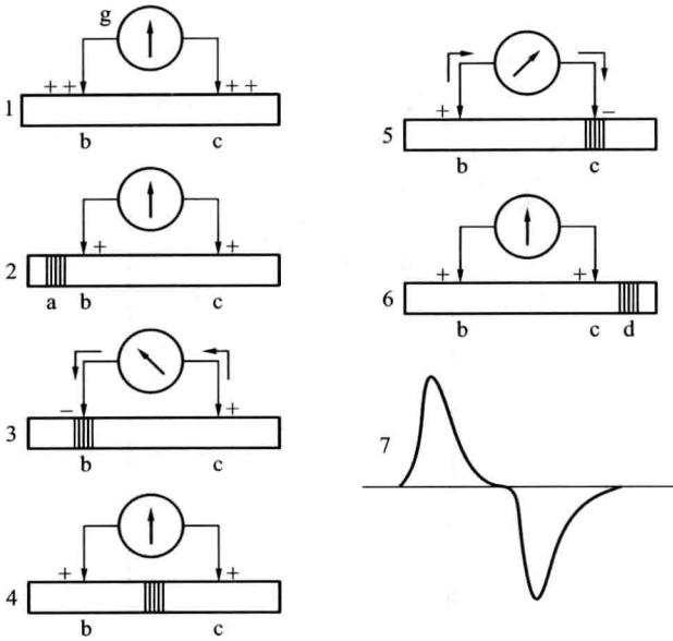
图 13.3 神经干上的动作电位示意图
