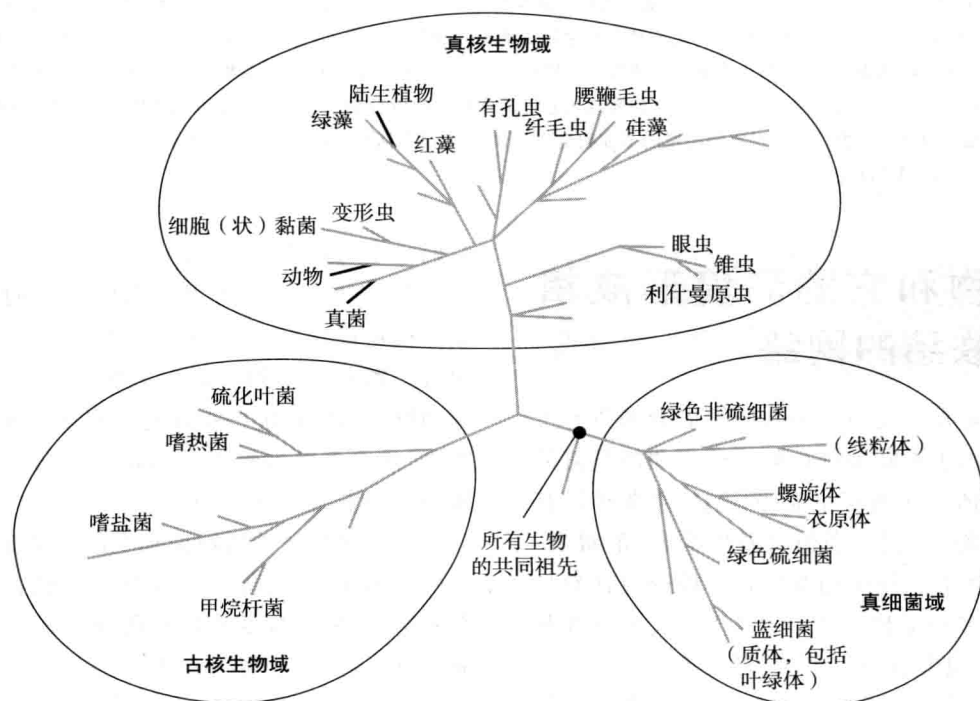
图 1.3 生命进化的三域学说 (引自 Reece, 2011) 这里的系统发生树是根据 rRNA 序列绘制的。分支的长度是同各个谱系遗传变化的数量成比例的。为了简化, 本图仅仅标志了某些分支。在真核生物域, 多细胞生物占优势的谱系有植物、真菌和动物, 所有其他谱系主要由单细胞生物组成。
