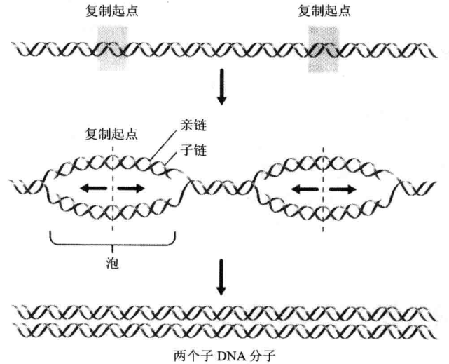
图 21.6 真核生物 DNA 复制中的多泡现象(引自坎贝尔等 2006)
