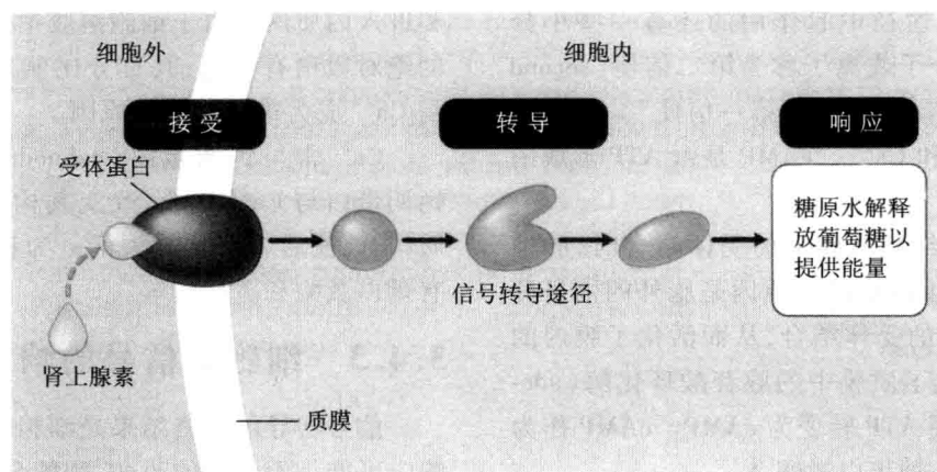
图 3.32 细胞信号转导途径(引自坎贝尔等,2006) 肾上腺素引起肌肉细胞中糖原的水解。
