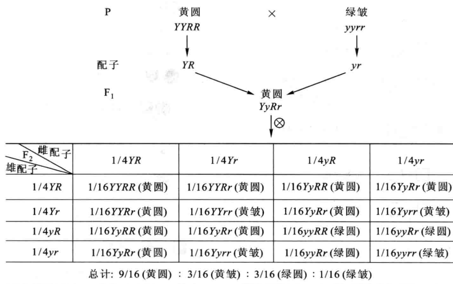
图 20.2 豌豆两对性状的自由组合 设:Y代表黄色基因,R代表圆形基因,y和r分别代表它们的隐性等位基因。
