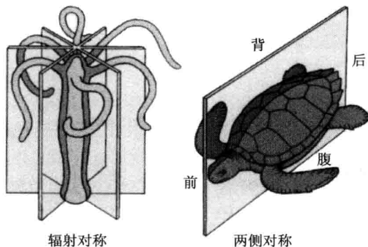
图32.1 辐射对称(水螅)与两侧对称(海龟)(仿自 Mader, 2001)
