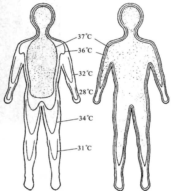
图10.2 人体的体壳温度与体核温度(仿自 Schmidt-Nielsen, 1979)
