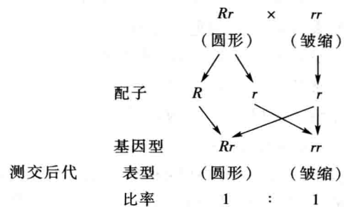
图 20.1 豌豆种子形状的分和孟德尔的假设
