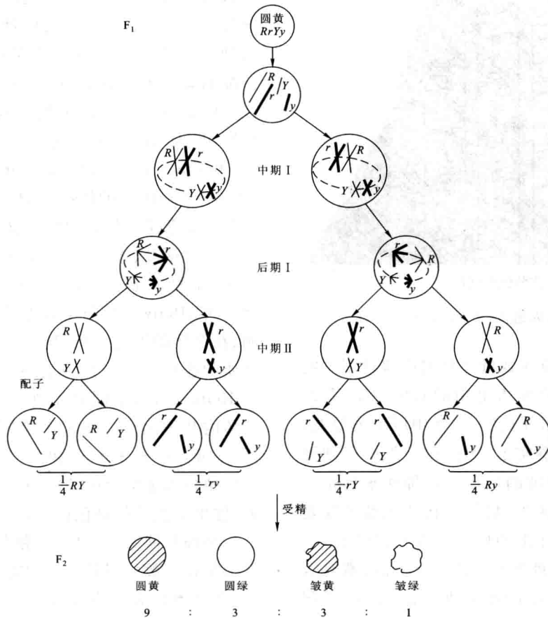
图 20.7 遗传的染色体学说示意图(改绘自 Campbell 等, 1997)
