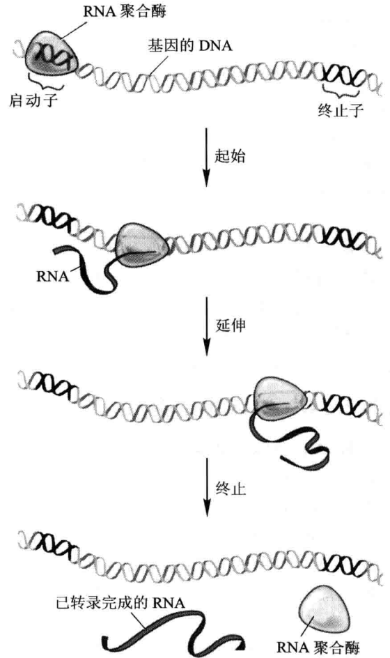
图 21.9 一个基因转录的 3 个步骤 (改绘自 Campbell 等,1997)
