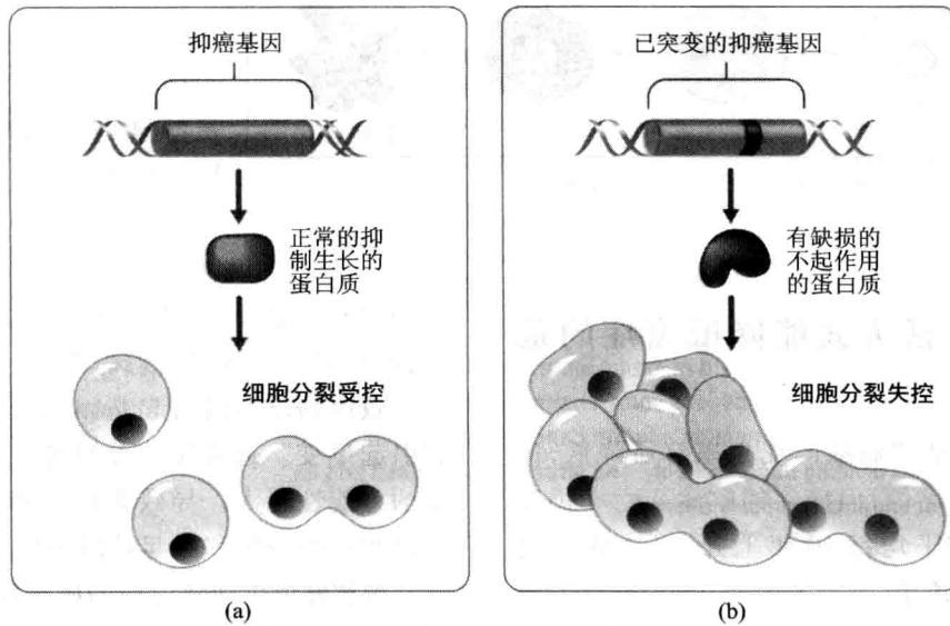
图 24.8 抑癌基因(引自吴相钰,2006) (a) 正常情况下编码一种抑制细胞生长和分裂的蛋白质。这时此基因有助于阻止癌细胞的出现。(b) 当抑癌基因中的突变使其蛋白质有缺损时,通常在正常蛋白质控制之下的细胞可能分裂过盛,最终形成癌。
