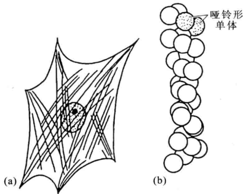
图 3.19 微丝 (a) 小鼠成纤维细胞中的微丝。(b) 哑铃形单体纤维。
