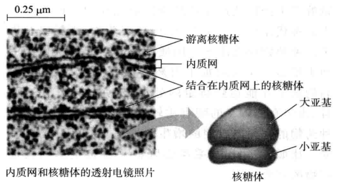
图 3.9 核糖体(引自 Reece, 2011)
