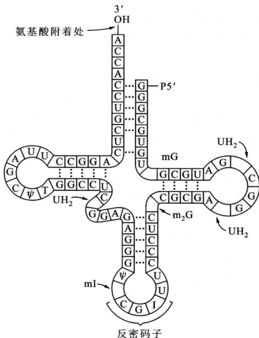
图 21.7 tRNA 结构和反密码子
