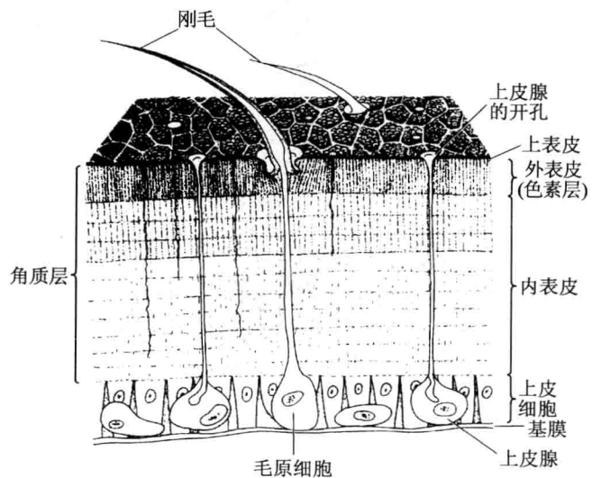
图 32.15 节肢动物的外骨骼 (仿自 Hackman,1971)
