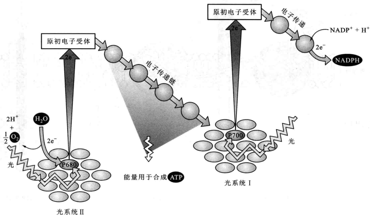
图 4.26 光合电子传递链
