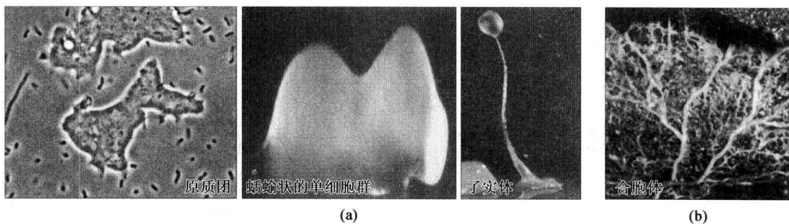
图 29.6 黏菌(引自 Campbell 等,1997) (a)盘基网柄菌(细胞型黏菌)。(b)原质型黏菌。
