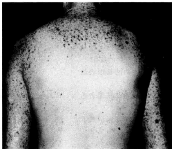
图 21.19 皮肤癌患者背面(引自 Griffiths 等,2000) 黑色斑点区示背部双肩及两臂皮肤癌变。
