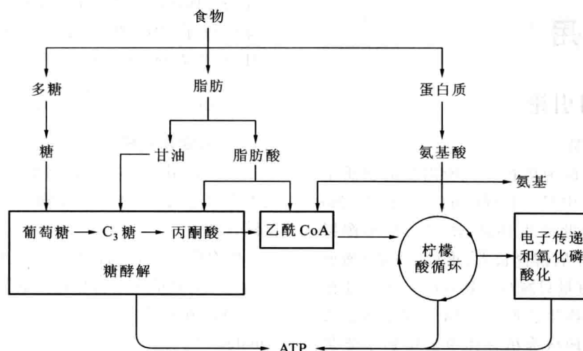
图 4.20 各种食物分子的分解
