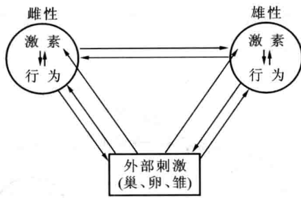
图 39.13 环鸽的激素、行为与环境三者之间的关系 双向箭头表示反馈关系,单向箭头表示直接影响
