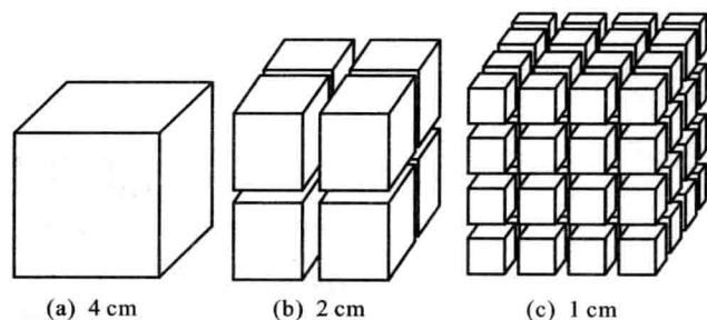
图 3.2 体积与面积的关系 (a) 表面积为 96 \text{ cm}^2 , 体积为 64 \text{ cm}^3 , 表面积: 体积为 1.5:1 。(b) 表面积为 192 \text{ cm}^2 , 体积为 64 \text{ cm}^3 , 表面积: 体积为 3:1 。(c) 表面积为 384 \text{ cm}^2 , 体积为 64 \text{ cm}^3 , 表面积: 体积为 6:1 。
