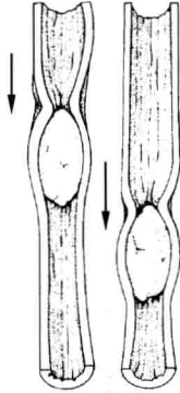
图 7.5 食管的蠕动(仿自 Eckert,1983)
