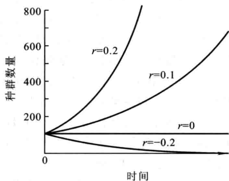
图 35.6 种群起始数量为 100 时,具有不同 r 值种群的数量动态(改绘自 Hedrick, 1984)
