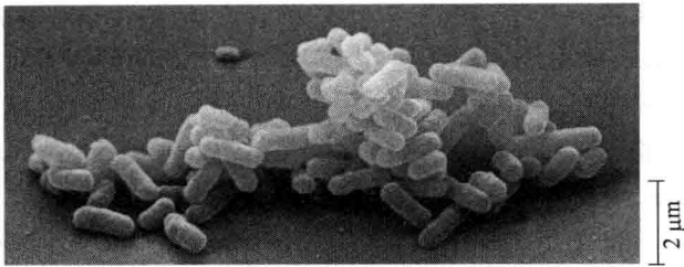
(a)真细菌域
