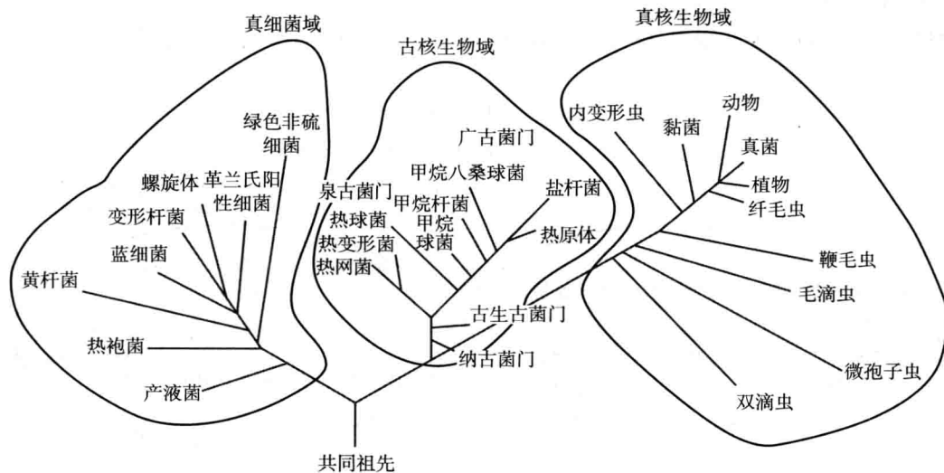
图 28.10 生命系统树 (Olsen 和 Woese, 1993) (仿自 Campbell 等, 2011)
