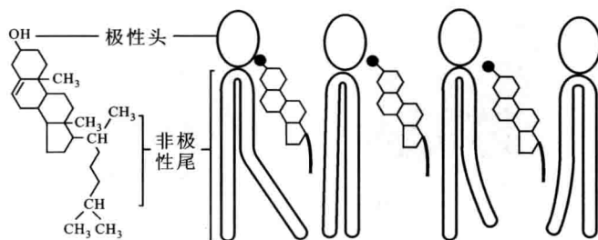
图 3.29 磷脂分子层中的胆固醇
