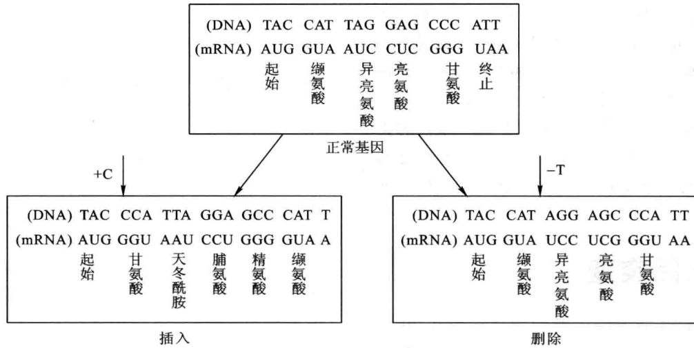
图 21.17 插入及删除引起的突变
