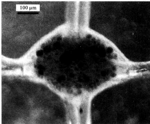
中华金钱蛭的神经节 (张人骥提供)
