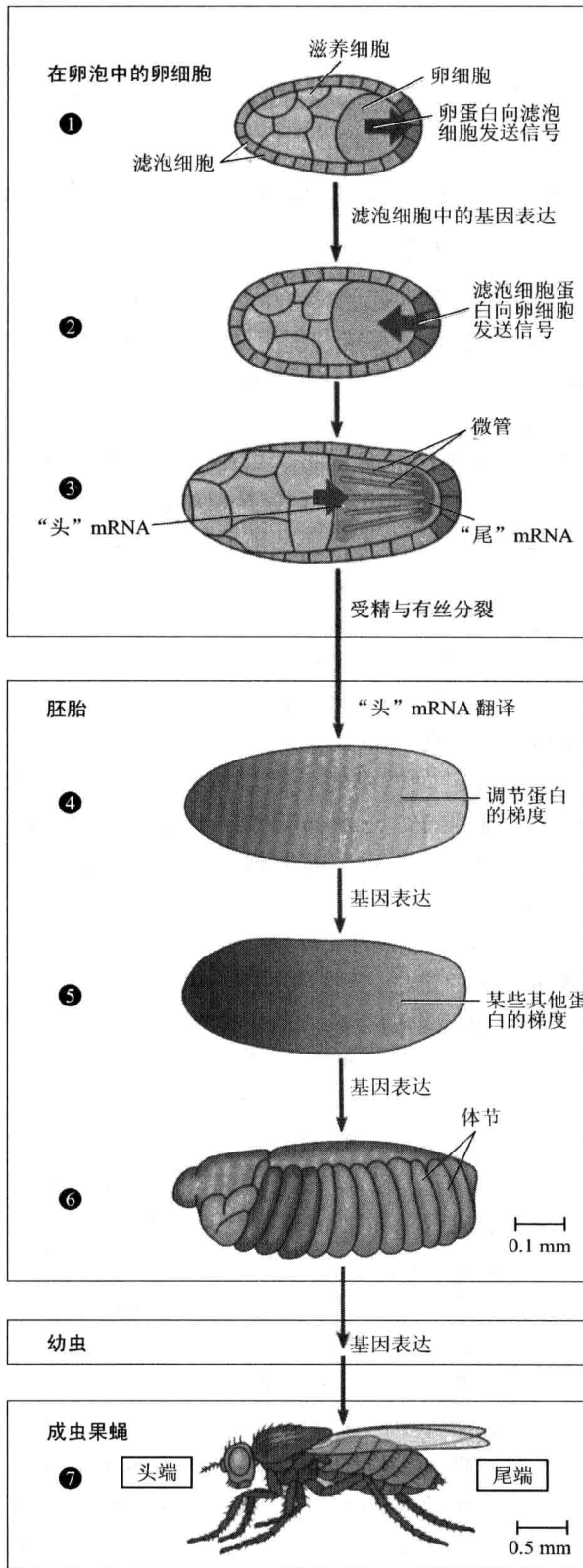
图 22.11 果蝇前后轴早期发育的关键阶段(引自 Campbell 等,1997)
