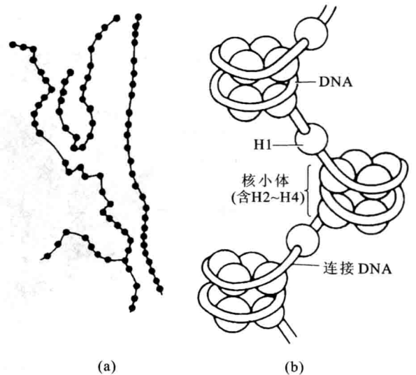
图 3.7 核小体 (a) 根据电镜观察结果而绘制的高度伸展的染色质示意图。(b) 核小体结构示意图。
