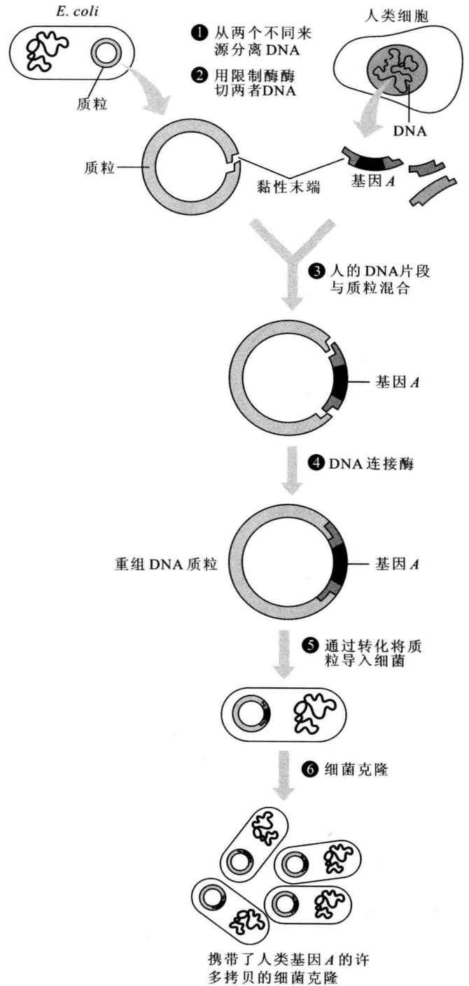
图 23.5 在细菌质粒中克隆基因(引自 Campbell 等,1997)
