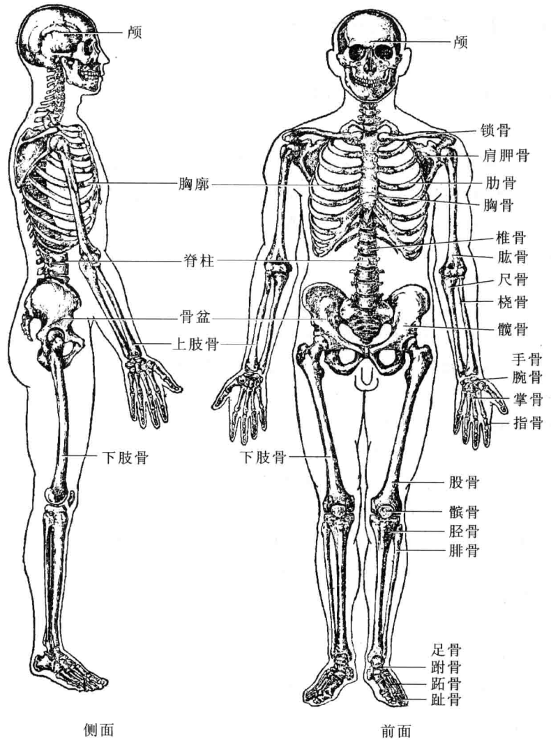
图 15.3 人体的骨骼系统(引自北京师范大学等,1981)
