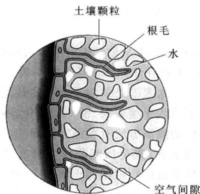
图 18.5 土壤中的根毛
