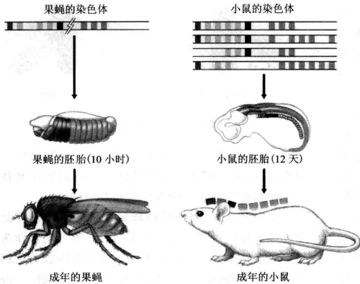
图 22.15 两种不同动物中的同源异形基因 图中最上方是果蝇和小鼠的染色体中携带同源异形基因的部分。其中各种不同灰度的小方块代表果蝇和小鼠的非常近似的同源异形基因(DNA 序列特别相近)。以下的同样花纹表示这些动物体内由这些基因所控制的部分(引自 Campbell 等, 2004)
