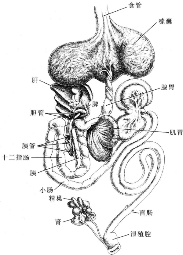
图 32.35 鸽的消化系统(仿自 Kent,1987)
