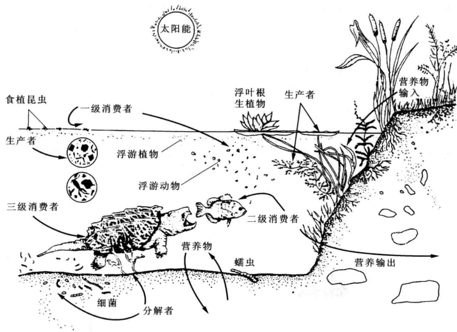
一个池塘生态系统(引自 Stiling, 1999)
