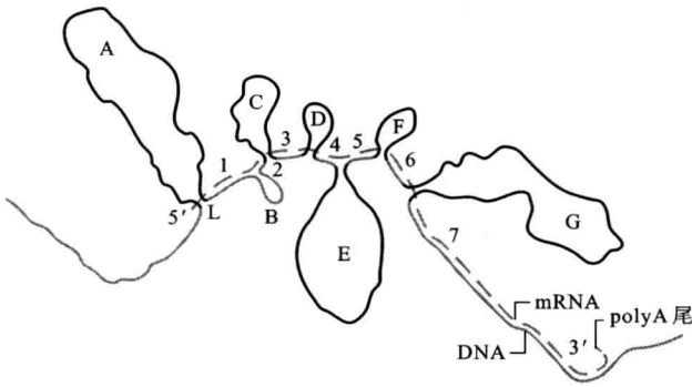
图 22.8 断裂基因 鸡的卵清蛋白基因, A~G 为内含子, 1~7 为外显子
