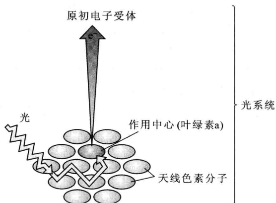
图 4.25 光系统中能量的传递和作用中心中叶绿素 a 的激发(改绘自 Campbell 等, 2000)
