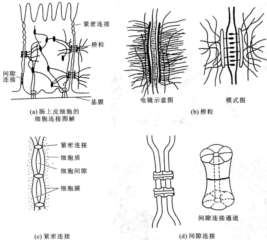
图 3.25 动物细胞的细胞连接
