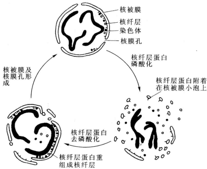
图 5.5 有丝分裂时核被膜的解体和再生
