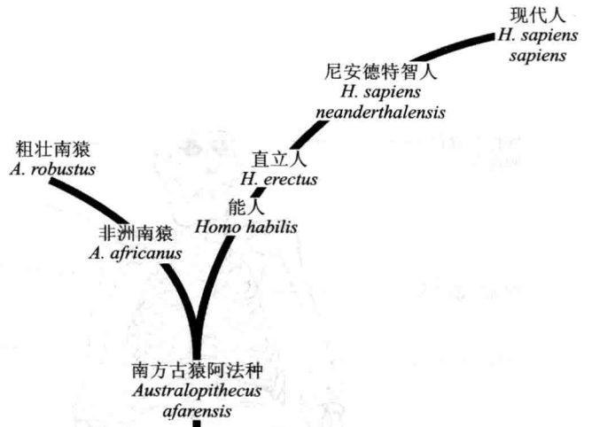
图 33.5 人亚科直线进化图解
