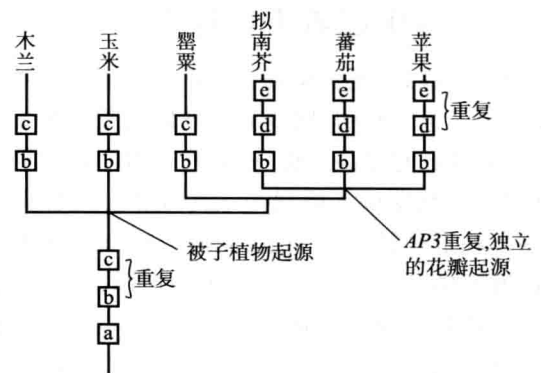
图 27.13 通过基因重复而实现的花瓣的进化 图示在被子植物起源之前, MADS box 基因经重复产生了 PI 和 PaleoAP3 基因。包括苹果、番茄、拟南芥等物种在内的进化支在和罂粟科产生分歧形成不同分支以后, PaleoAP3 重复产生了 AP3 和 AP3 重复。实验证明, AP3 具有控制花瓣发育的功能。a: 祖先基因, b: PI , c: PaleoAP3 , d: AP3 , e: AP3 重复。
