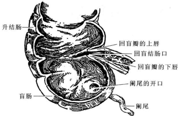
图 7.10 回盲瓣的构型(引自北京师范大学等,1981)
