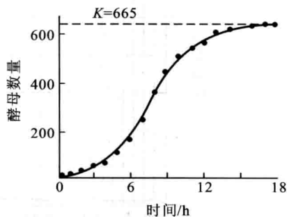
图 35.8 酵母种群的逻辑斯谛增长
