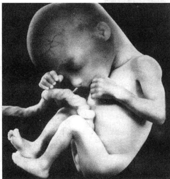
16 周的胎儿(引自 DeWitt, 1989)
