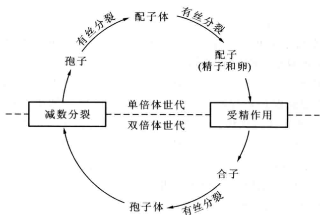
图 30.1 植物的世代交替图解
