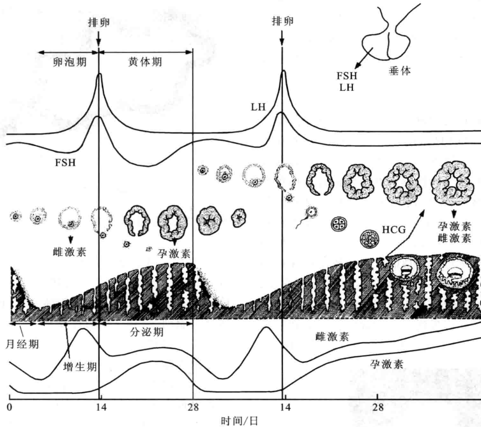
图 16.13 卵巢周期与子宫周期(仿自 McNaught)
