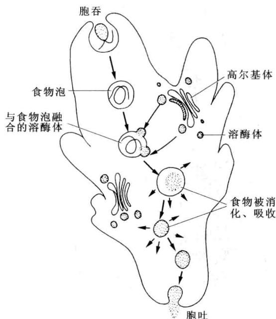
图 3.12 溶酶体参与细胞消化
