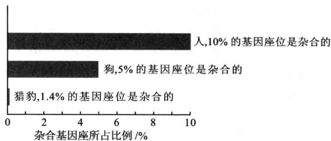
图 25.8 猎豹的遗传变异比人和狗的小得多
