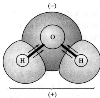
图 2.1 水分子的极性(仿 Campbell 等,1999)
