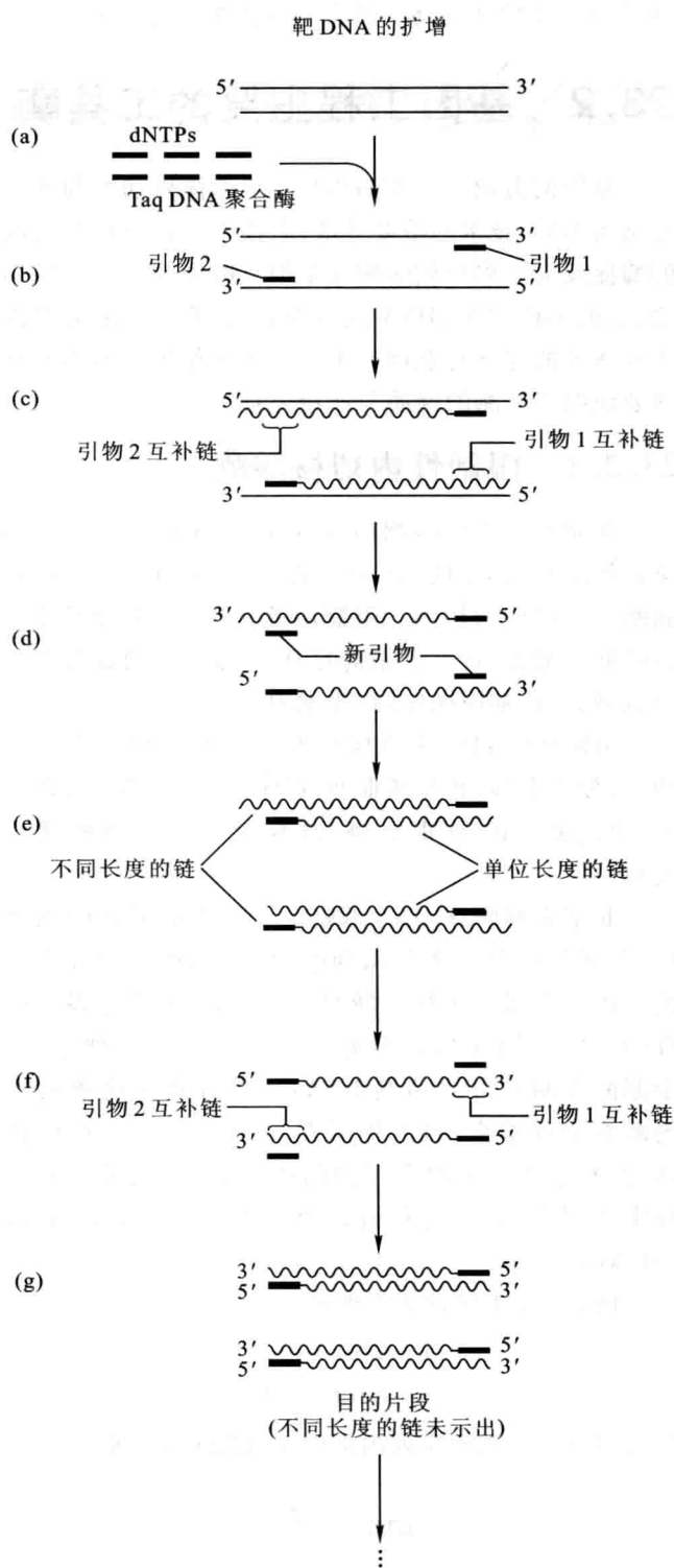
图 23.2 PCR 反应示意图 (改绘自吴乃虎, 1998)
