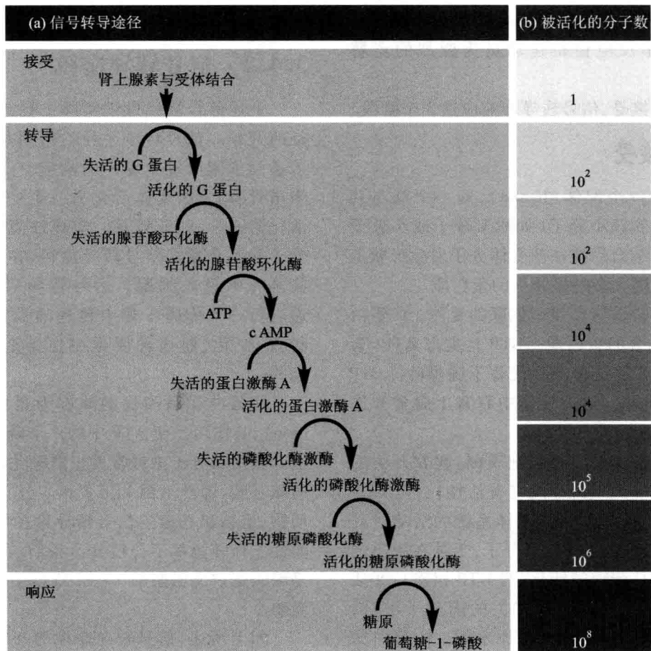
图 3.33 细胞对信号的响应(仿 Campbell 等,2002) 肾上腺素引起糖原的降解。
