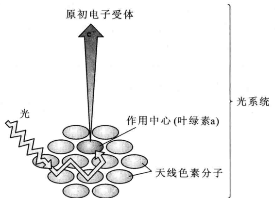
图 4.25 光系统中能量的传递和作用中心中叶绿素 a 的激发(改绘自 Campbell 等, 2000)
