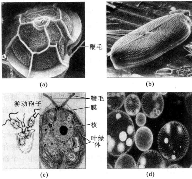
图 29.3 单细胞或群体藻类(引自 Campbell 等,1996) (a) 沟鞭藻。(b) 硅藻。(c) 衣藻。(d) 团藻。
