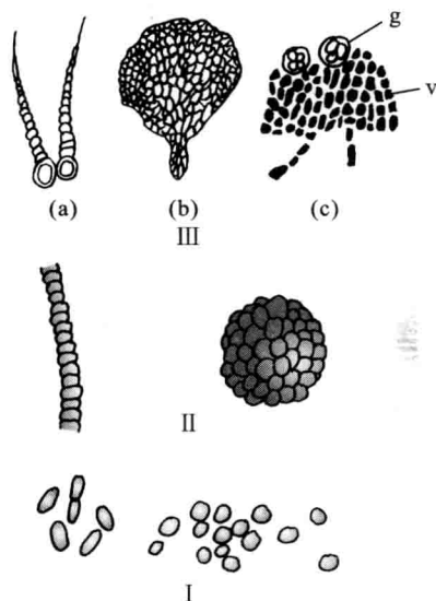
元古宙原核生物蓝细菌的多细胞化趋势(张昀根据河北庞家堡长城群蓝细菌化石的研究资料绘制)由单个细胞(I)到非极性集群(II),发展到有两极(上部和下部)分化的极性集群(III a,b),以及有生殖细胞(g)和营养细胞(v)分化的极性集群(III c)。
