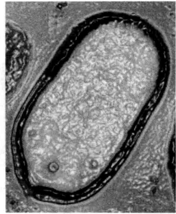
图 28.14 潘多拉病毒颗粒的电子显微镜图像 (引自《科学》2013 年第 341 卷第 6143 期封面图)
