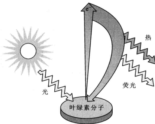
图 4.24 溶液中叶绿素发出荧光(改绘自 Campbell 等, 2000)
