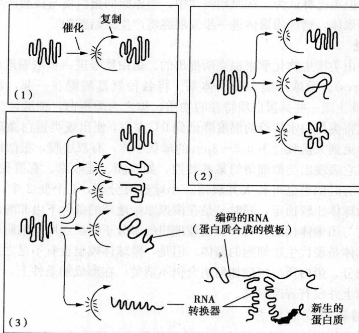
图 17-2 指导蛋白质合成的 RNA 自我复制系统在进化中的三个相继阶段 (引自 B. Alberts 等, 1989 年)
