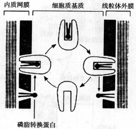
图 7-15 磷脂转换蛋白转移磷脂示意图
