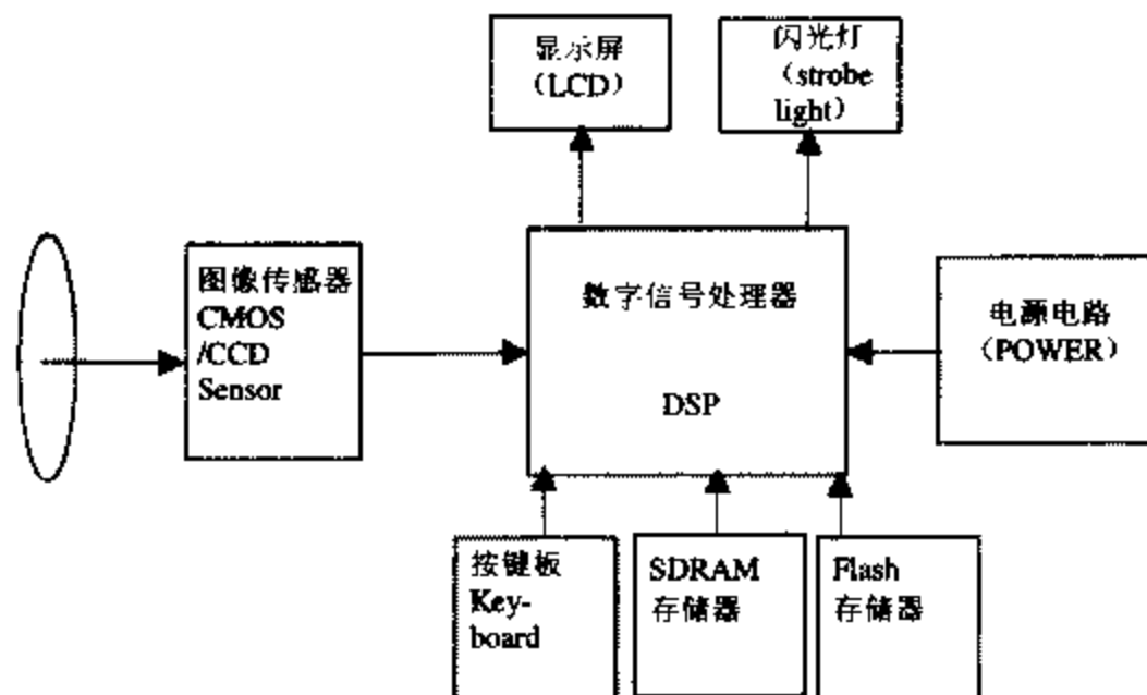
图7-38 数码相机的组成
